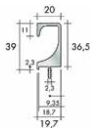
Greeplijst type 900303
